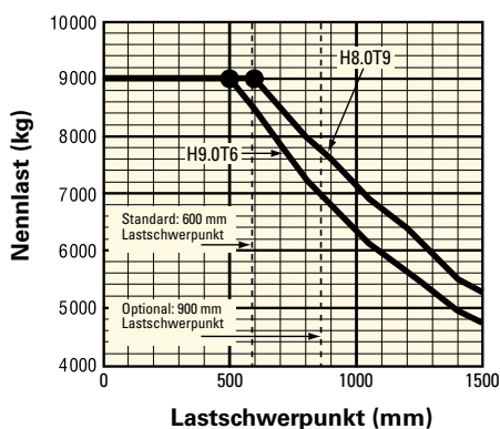
GABELTRÄGER FÜR HAKENGEFÜHRTE GABELZINKEN MIT INTEGRIERTEM SEITENSCHIEBER
