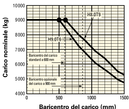
PIASTRA PORTAFORCHE AD AGGANCIO CON TRASLATORE INTEGRATO E POSIZIONATORE FORCHE
