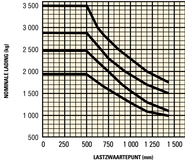
SIDESHIFT-VORKENBORD
