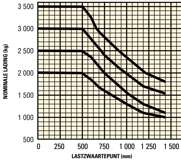
STANDAARDVORKENBORD
