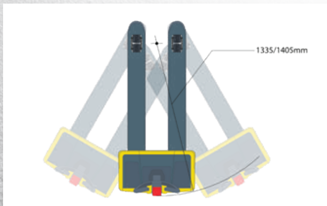
MINI Type Pallet Truck
